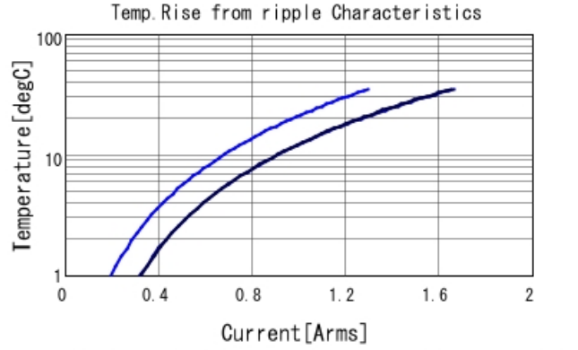
GRM188R72A104KA35 Temp. rise — 400kHz — 800I
